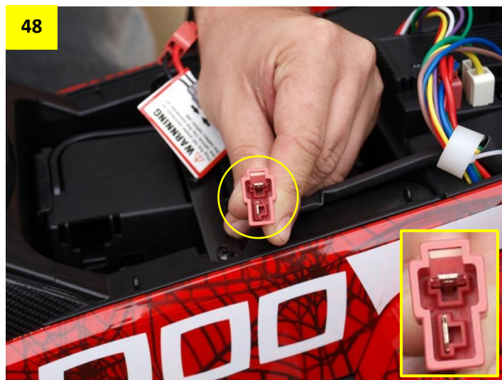
Obr. 48: Překontrolujte konektory pro zapojení baterie – mosazné packy v zástrčce musí být rovně a uprostřed. Jsou-li vychýlené ke stranám, narovnejte je prosím prstem.
