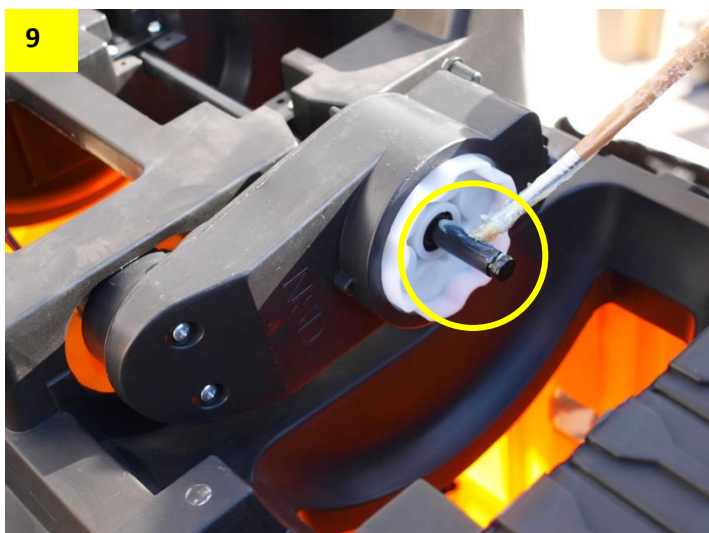
Obr. 10: Připravte si zadní kola.
